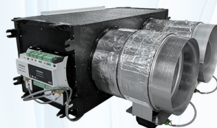
DN150
